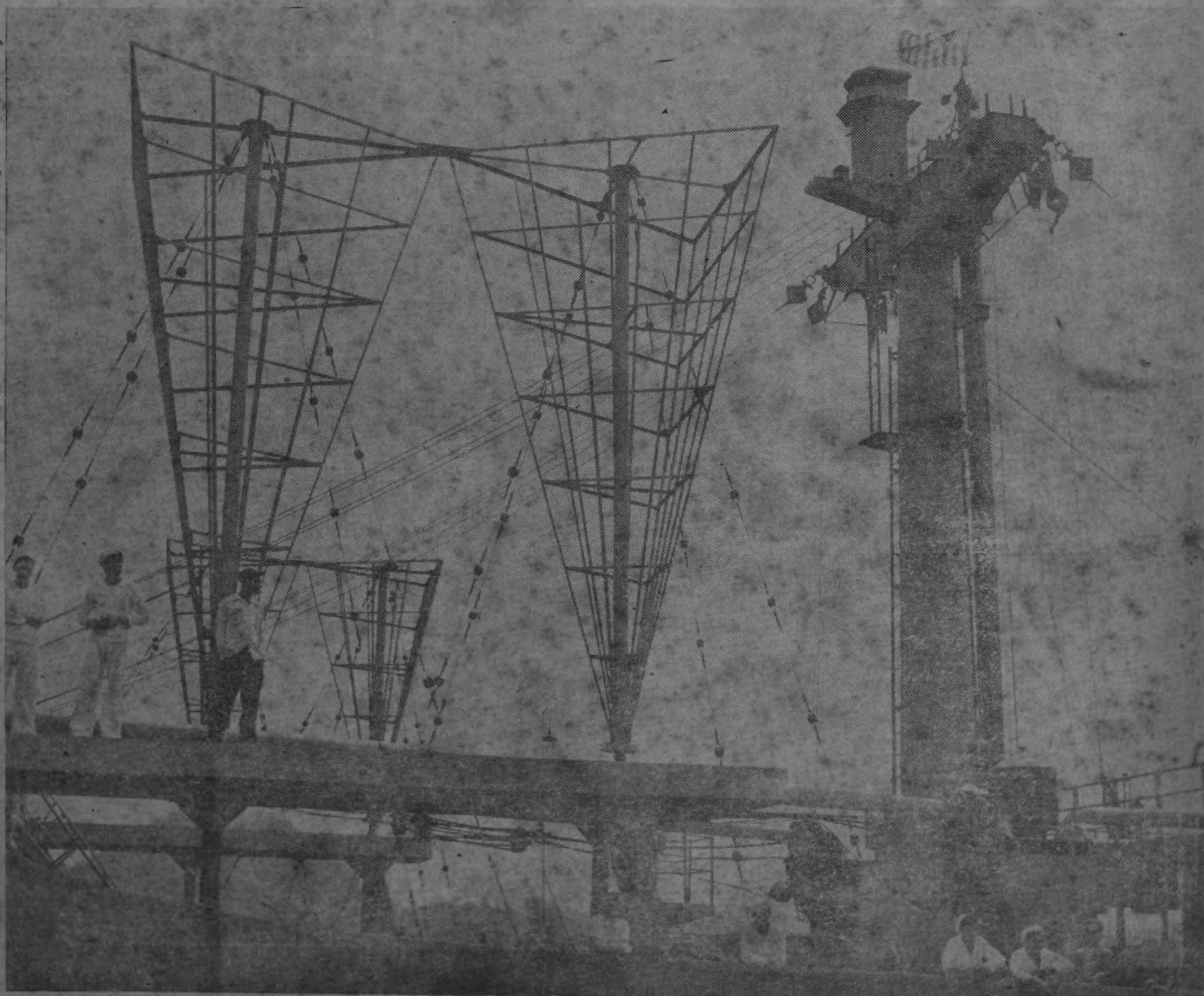
LAS ANTENAS DEL "COURIER". — Estas armazones de acero son las antenas de onda corta del "Courier", que trabaja con dos equipos trasmisores de 35.000 vatios cada uno. (Información sobre esta trasmisora errante de la verdad democrática.
